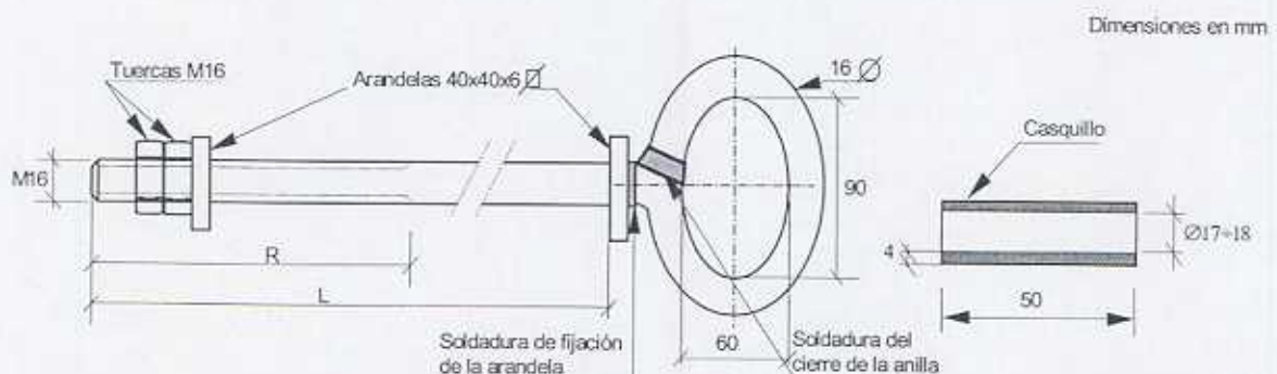
Figura 7 : Tornillo de anclaje para línea de seguridad TALS y casquillo para suplemento CS
