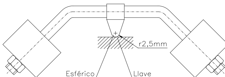
Fig. 4 – Aparato para el ensayo de la bola.
