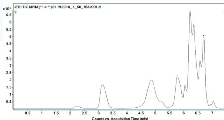
Cromatograma obtenido a partir de una muestra de aceite de oliva en el que se observa el perfil de compuestos fenólicos.
